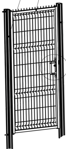
Рама 40х40мм
