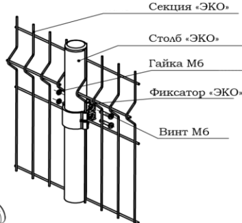
Монтажная схема
