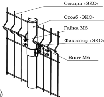
Монтажная схема
