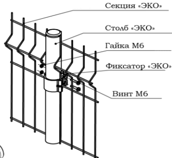
Монтажная схема
