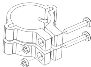
Столб 60х80мм
