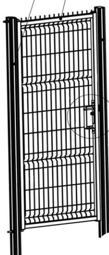
Столб 60x80мм Рама 40x40мм
