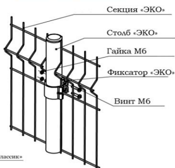
Монтажная схема
