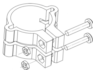
Столб 60х80мм
